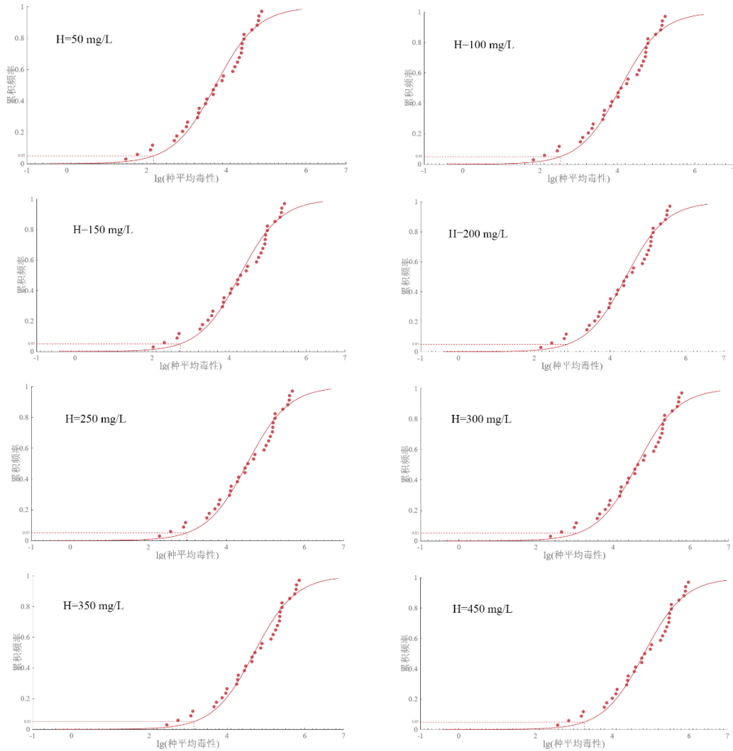
图 2 对数急性毒性—累积频率的逻辑斯谛分布模型拟合曲线 (H 为水体硬度)
