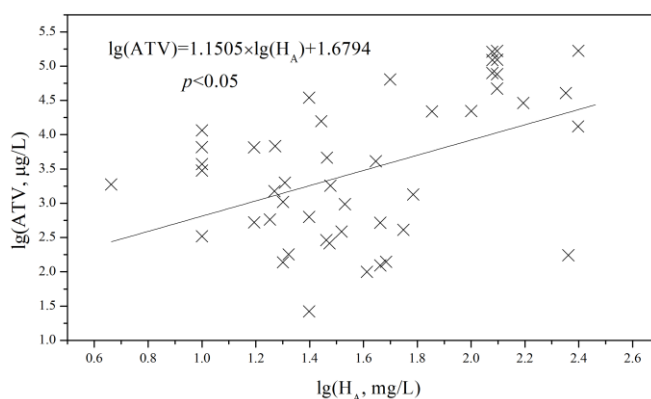
图 1 急性毒性值与水体硬度的线性关系
