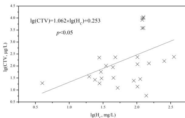
图 3 慢性毒性值与水体硬度的线性关系
