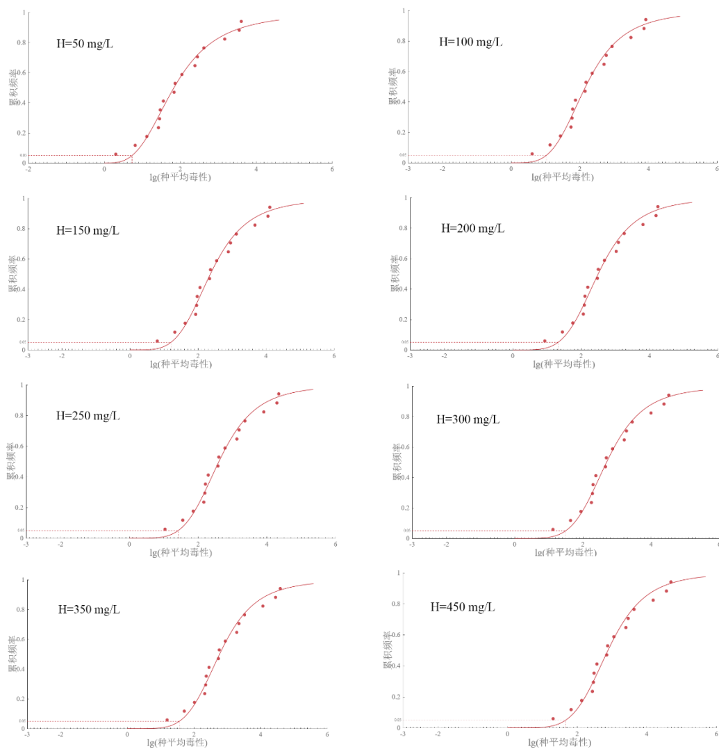
图 4 对数慢性毒性—累积频率的对数逻辑斯谛分布模型拟合曲线 (H 为水体硬度)
